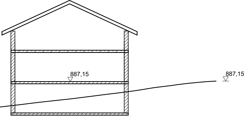
SCHEMASCHNITT G - G M 1 : 200
