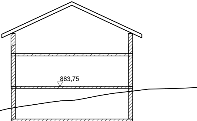
SCHEMASCHNITT I - I M 1 : 200
