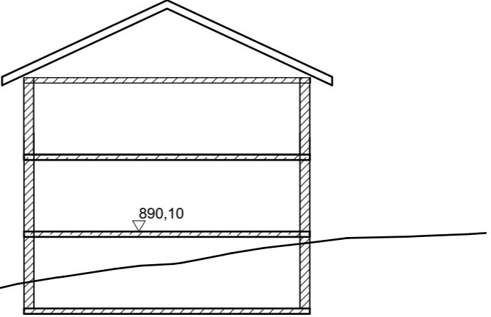
SCHEMASCHNITT J - J M 1 : 200
