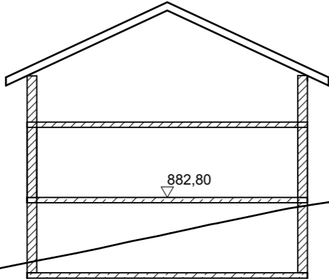
SCHEMASCHNITT F - F M 1 : 200
